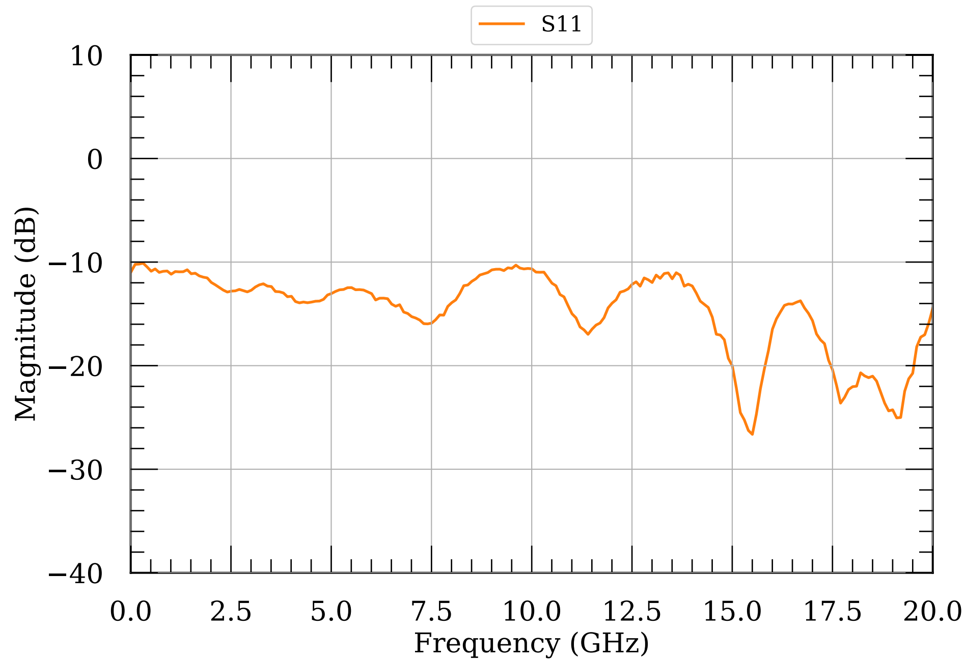
LNA S-params module092
